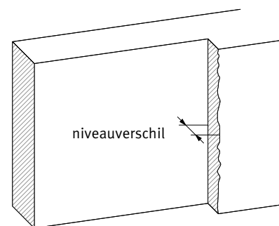
Afb. 143 Niveauverschil aan de buitenzijde van de ondergrond en tussen isolatieplaten.
