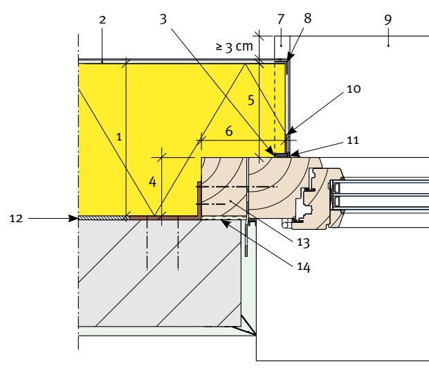
B. Horizontale doorsnede – Kader met stelkader
