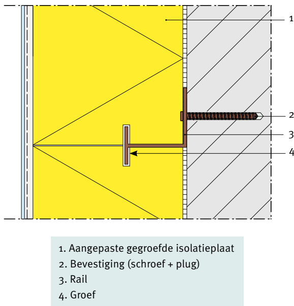
Afb. 21 Mechanische bevestiging op rails (doorsnede).
