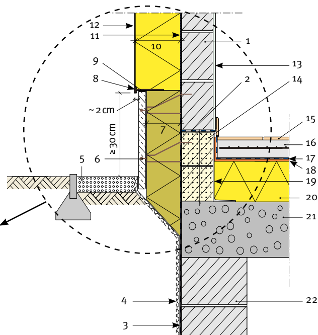
Afb. 48 Aansluiting aan de muurvoet met behulp van een isolerend bouwblok.
