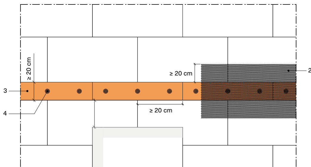
Afb. Cor.5 Brandwerend scherm (vooraanzicht).
