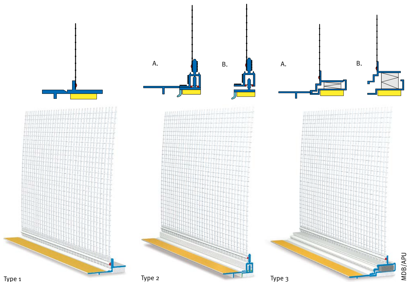
Afb. 34 Voorbeelden van profielen die de aansluiting verzekeren tussen de bepleistering en het schrijnwerk.
