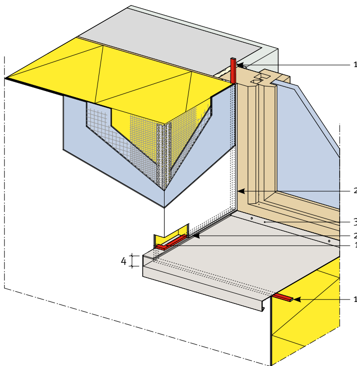
A. Metalen dorpel (3D)
