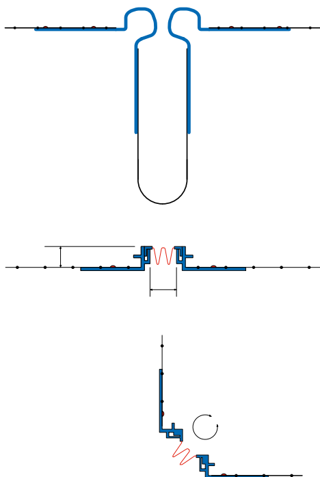
Afb. 35 Profielen voor bewegingsvoegen die uitgerust zijn met een soepele folie uit PVC (boven) of TPE (onder).
