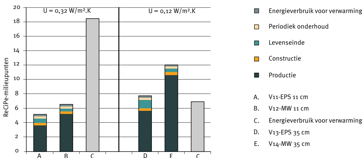
Afb. 41 Vergelijking van de milieu-impact tijdens de verschillende levenscyclusfasen (60 jaar) voor ETICS met EPS en rotswol, en U = 0,32 \text{ W/m}^2\text{K} of U = 0,12 \text{ W/m}^2\text{K} .
