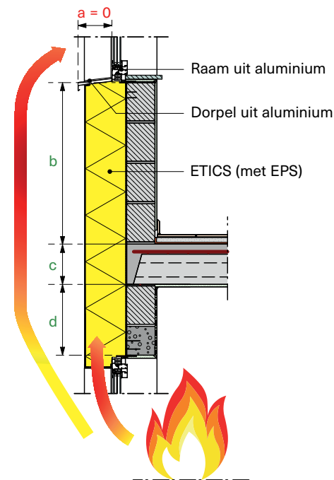
Afb. Cor.1 Ontwikkelde lengte van 1 m van het E60-element ( a + b + c + d ) ( a = 0 , vermits de dorpel uit aluminium en het ETICS geen E60 zijn).
