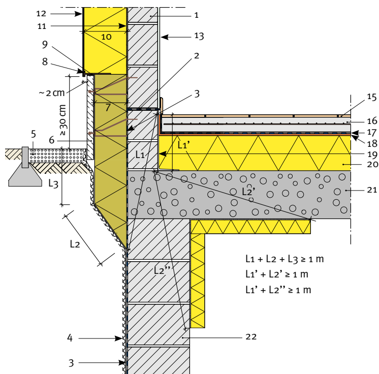
B. Op een niet-verwarmd aangrenzend volume (kelder, kruipruimte)
