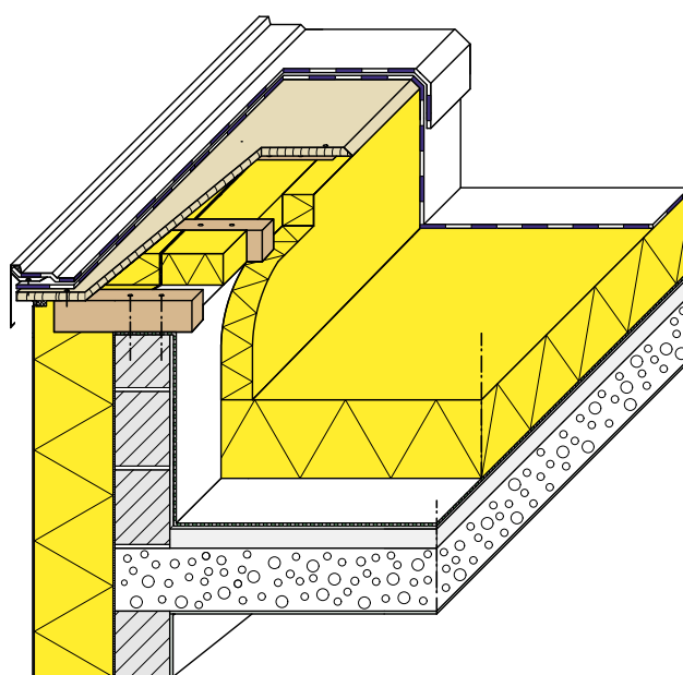
B. Doorsnede (3D)
