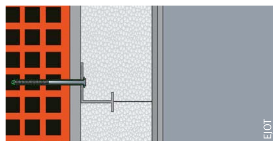
Afb. 120 Plaatsing van een rail of een profiel met behulp van een schroefplug (voorgemonteerde schroef).
