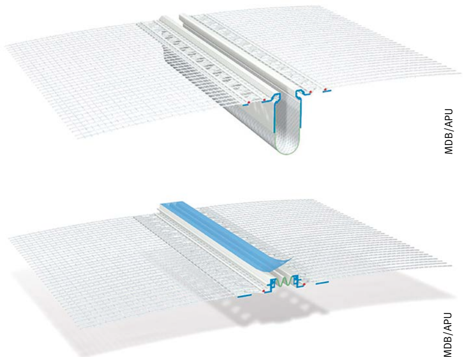
Afb. 35 Profielen voor bewegingsvoegen die uitgerust zijn met een soepele folie uit PVC (boven) of TPE (onder).
