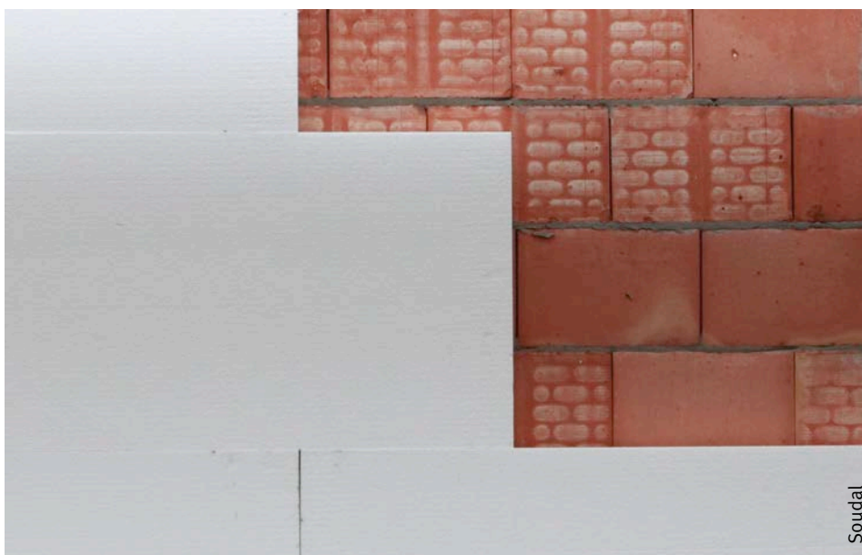
Afb. 99 Plaatsing die afgestemd is op de verspringende verticale voegen van platen met aangepaste dimensionale toleranties.
