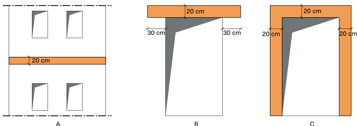
Afb. Cor.3 Soorten brandwerende schermen.
