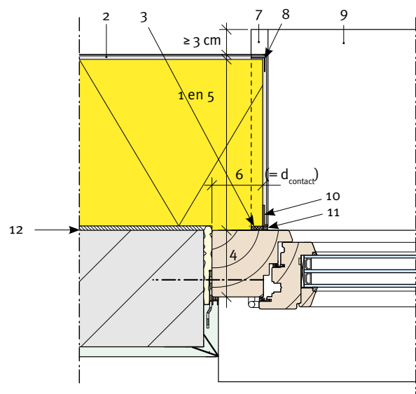
A. Horizontale doorsnede
