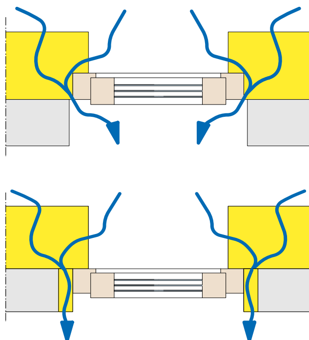
Afb. 38 Voorbeelden van geluidlekken ter hoogte van de aansluitingen met het ETICS.
