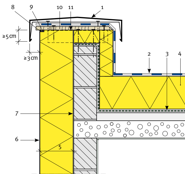
Afb. 68 Metalen muurkap.
