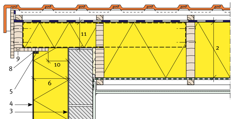
Afb. 76 Aansluiting van een ETICS met de dakzijrand (puntgevel) van een hellend dak.
