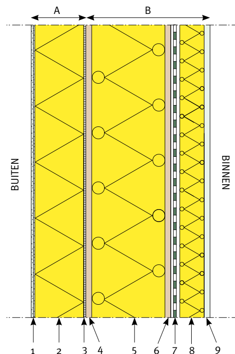
Afb. 43 Wand die opgebouwd is uit een ETICS op houtskelet: 3D (links) en 2D (rechts).
