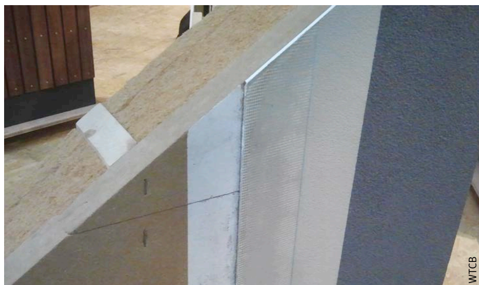
Afb. 24 Mechanische bevestiging van een isolatieplaat rechtstreeks op het skelet door middel van nieten.
