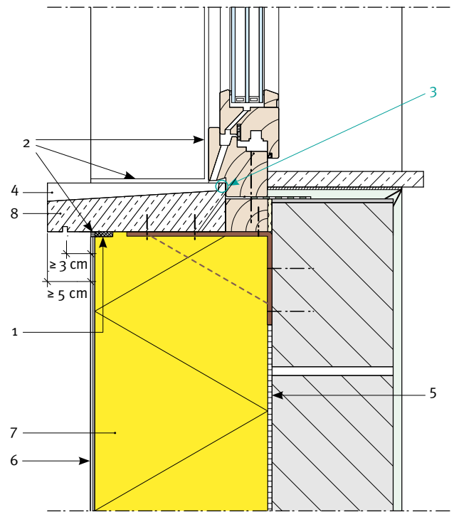
B. Natuurstenen dorpel (verticale doorsnede in 2D)
