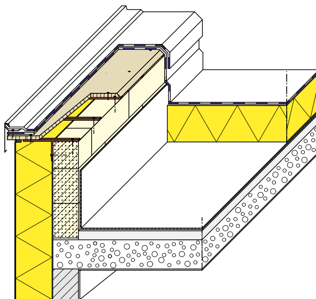
B. Doorsnede (3D)
