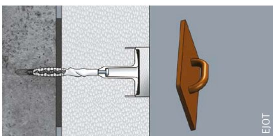
Afb. 118 Verzonken plaatsing van een schroefschotelplug (stalen schroef).
