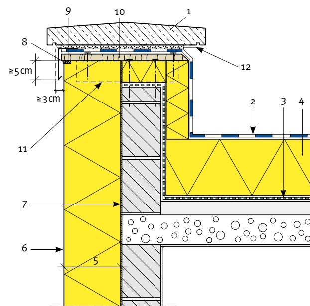
Afb. 69 Deksteen uit natuursteen of beton.
