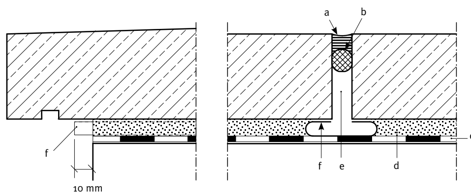
Afb. 70 Voegdetaillering bij dekstenen uit natuursteen of beton.
