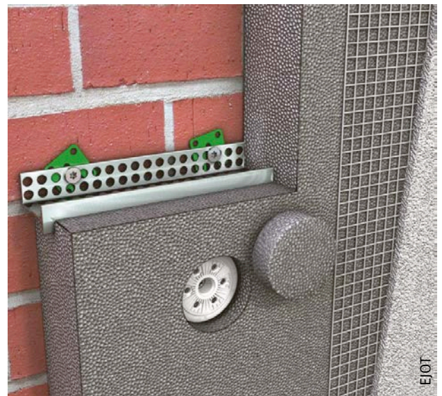
Afb. 22 Mechanische bevestiging op rails aangevuld met een schotelbevestiging.
