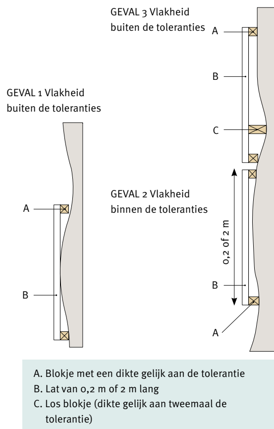
Afb. 138 Principe van de controle van de vlakheid.
