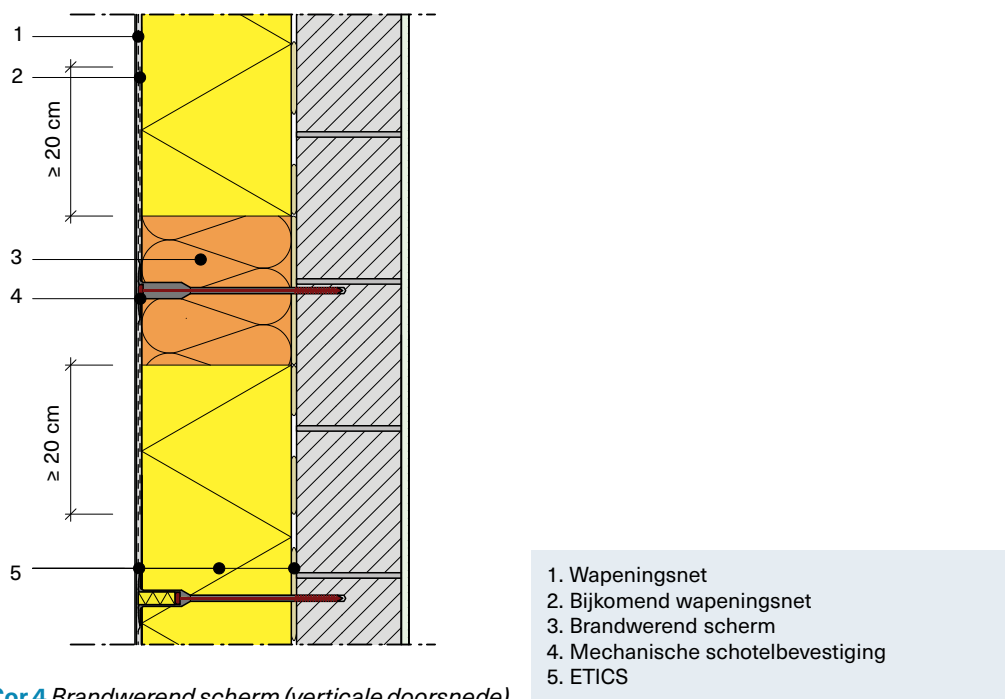
Afb. Cor.4 Brandwerend scherm (verticale doorsnede).
