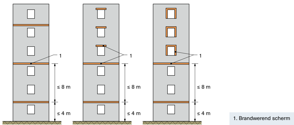
Afb. Cor.2 Typeoplossingen (brandwerende schermen) voor gevels van middelhoge gebouwen zonder een doorlopende luchtsponw.
